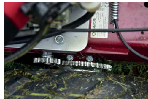
Mechanická uzávěrka diferenciálu je složená z pastorku a ozubeného kola. Vypíná se zpravidla při otáčení stroje na souvrátí
